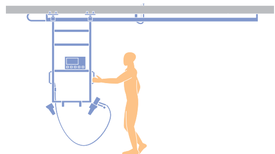
Lösung mit Werkzeugablage
