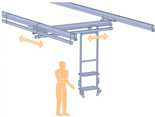
X-Y-Anwendung mit Energieführung. Luft- und Stromversorgung ohne Spiralschläuche oder Kabelschlaufen.
