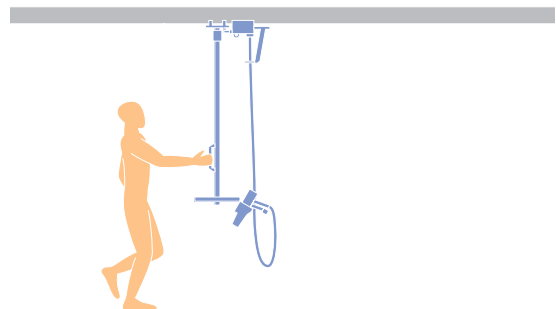
Lösung mit Abnahmewagen und Werkzeuggehänge
