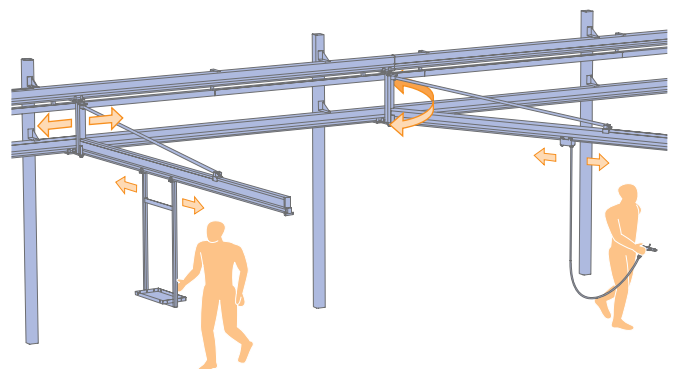
Schwenkausleger in einer Linie
